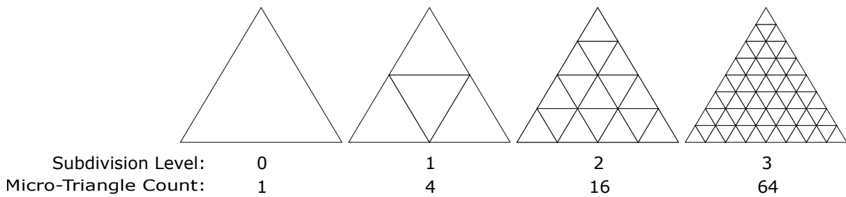
Fig. 5.1 - Microtriangle subdivision
