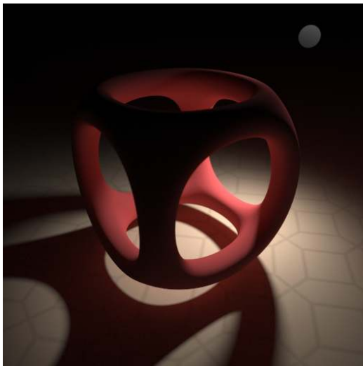
Fig. 5.9 - spot_edf
