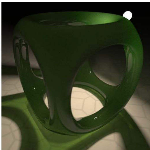
Fig. 5.13 - anisotropic_vdf
