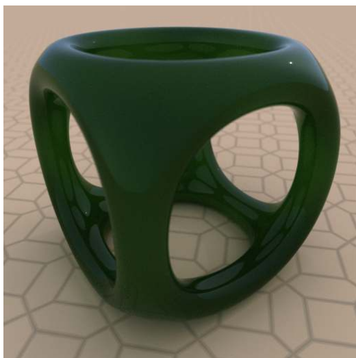
Fig. 5.12 - anisotropic_vdf
