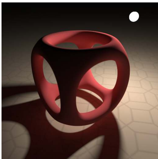
Fig. 5.8 - diffuse_edf
