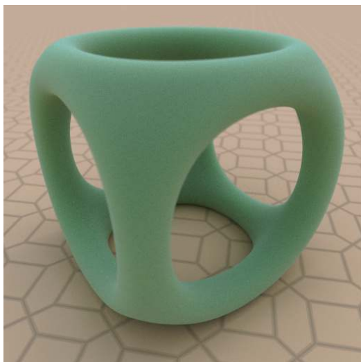
Fig. 5.11 - anisotropic_vdf
