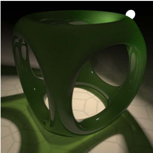
Fig. 5.13 - anisotropic_vdf
